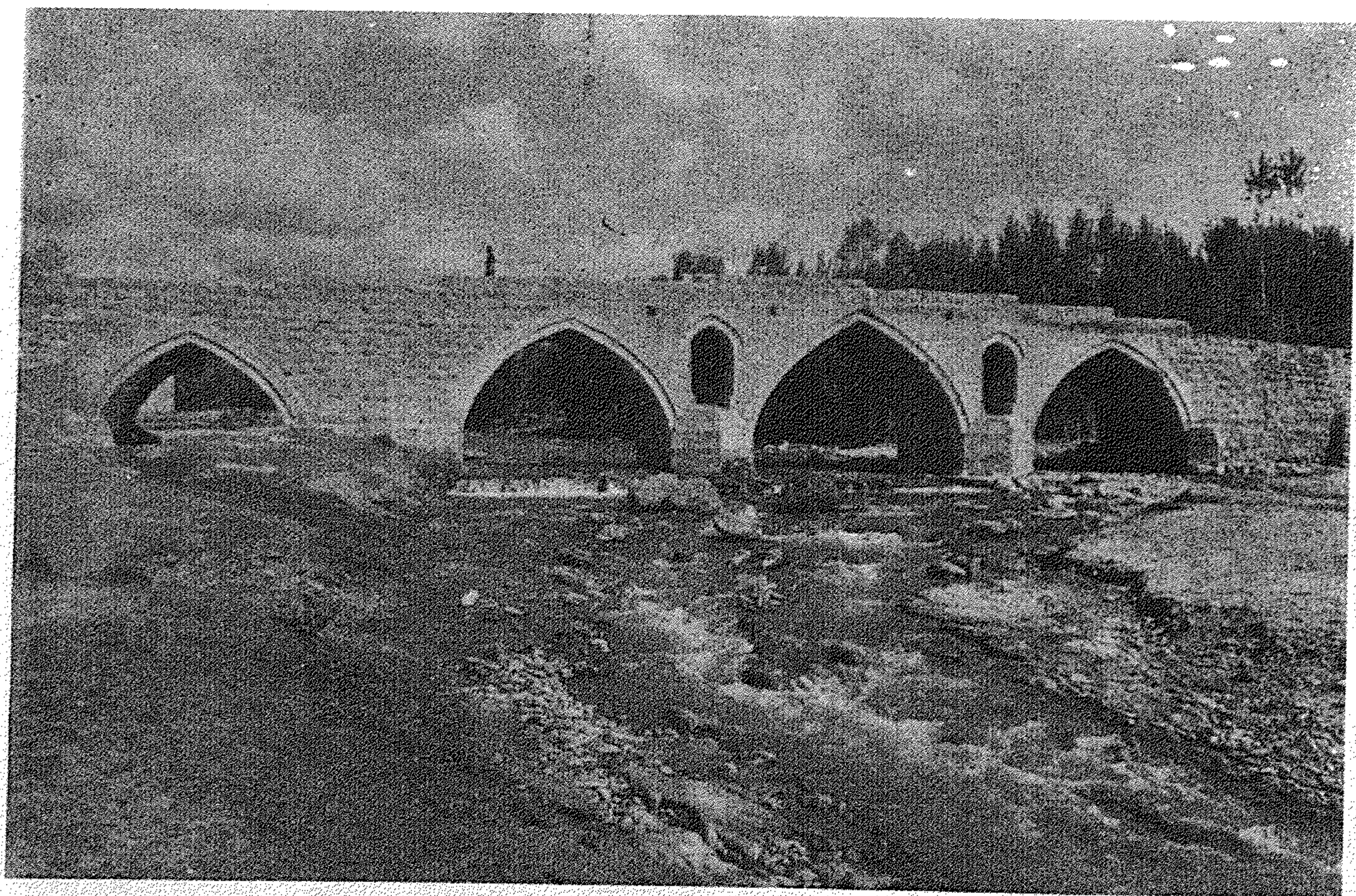
۷۷- پل دختر در قافلانکوه در هنگام آبادی
